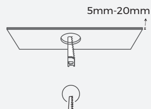
开孔尺寸: φ75mm
